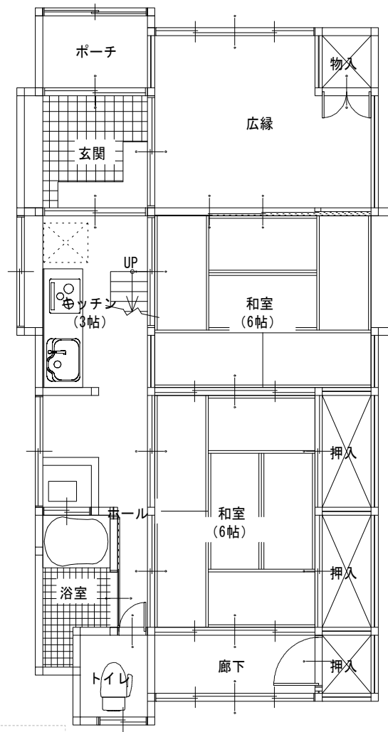
住宅 1 F 平面図
